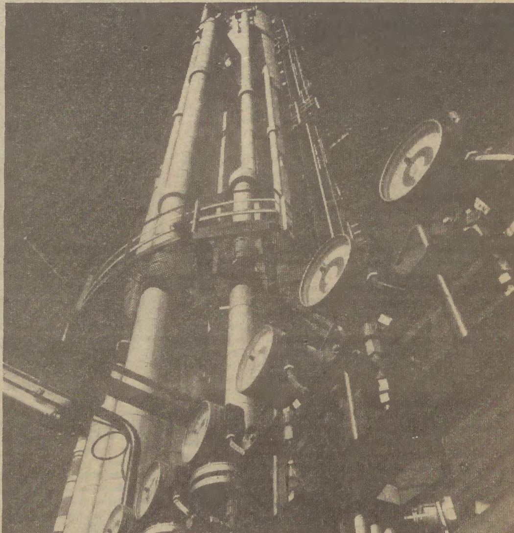
Os trabalhadores consideram positivas as acções de reestruturação que não levam ao desmembramento da Quimigal. Na foto: unidade 450 de descarbonatação da Fábrica de Amoníaco do Lavradio (Quimigal, EP)
